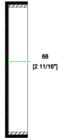
A-A VIEW
