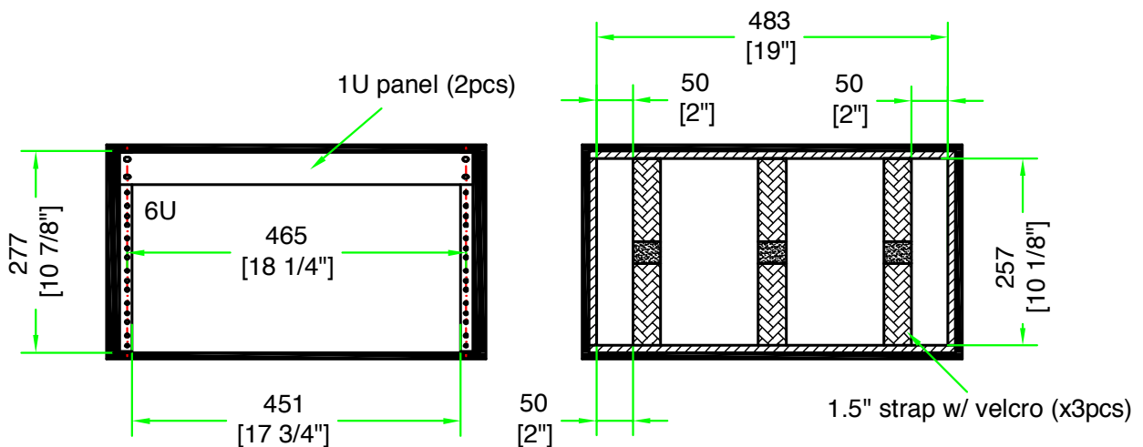
A-A VIEW
