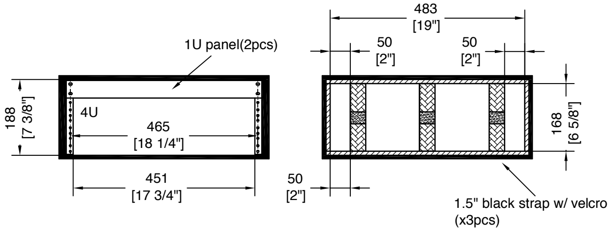
A-A VIEW
