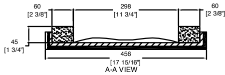
A-A VIEW
