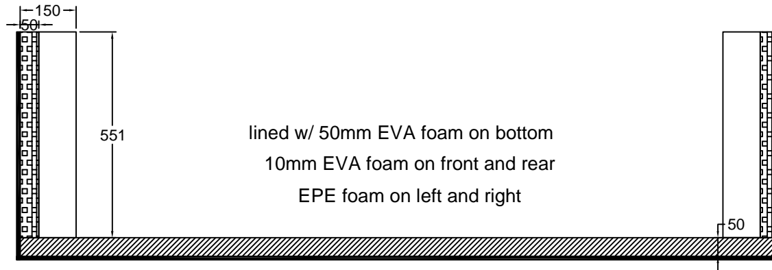
A-A VIEW
